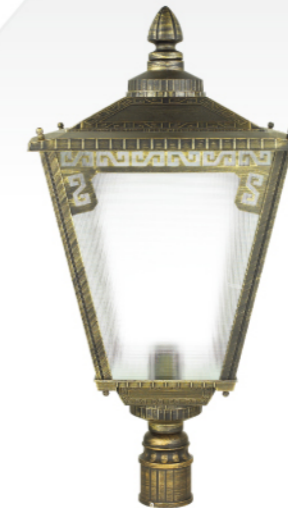
4240-3 L W H 400 400 770
